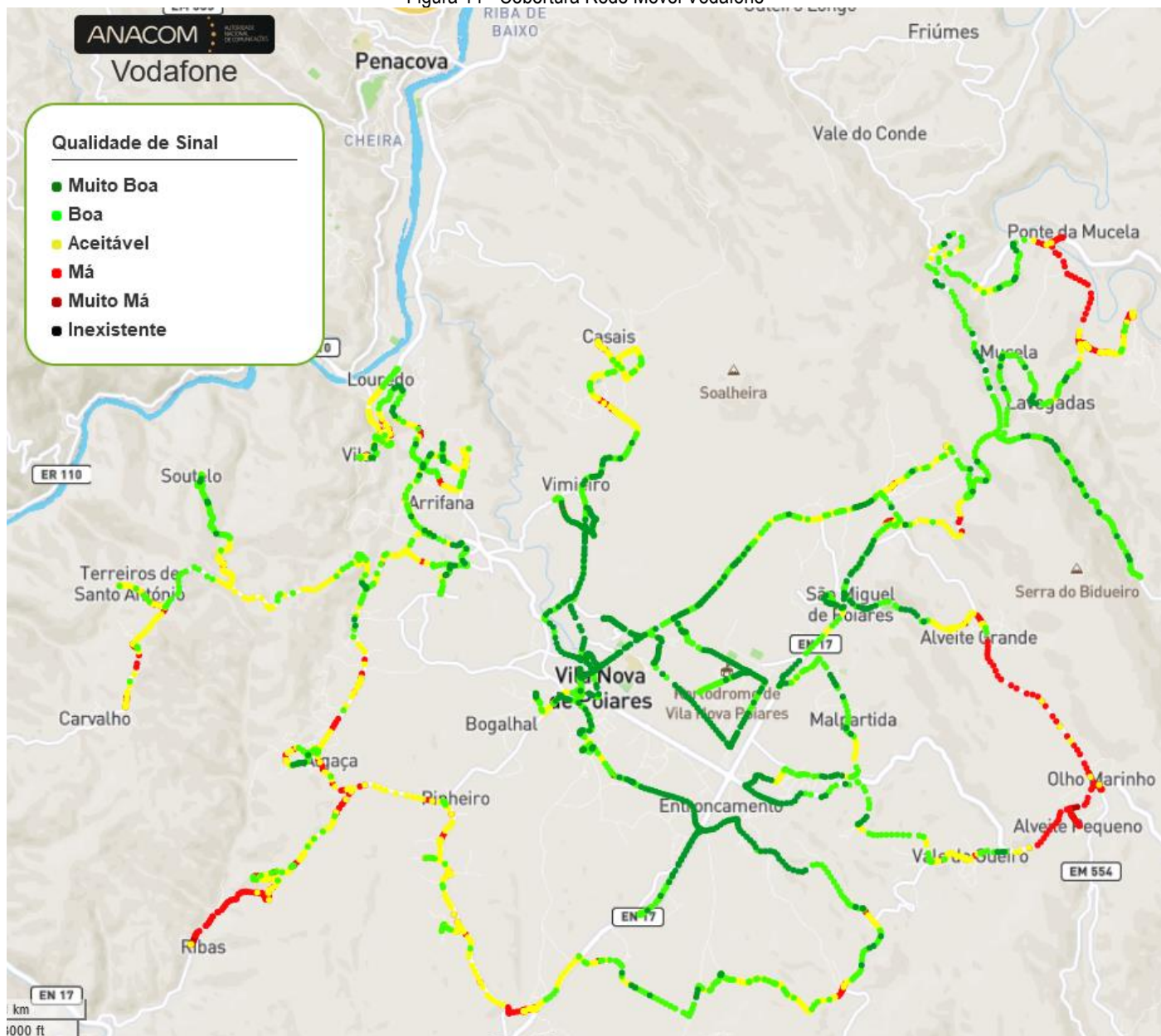
Figura 14 - Cobertura Rede Móvel Vodafone
