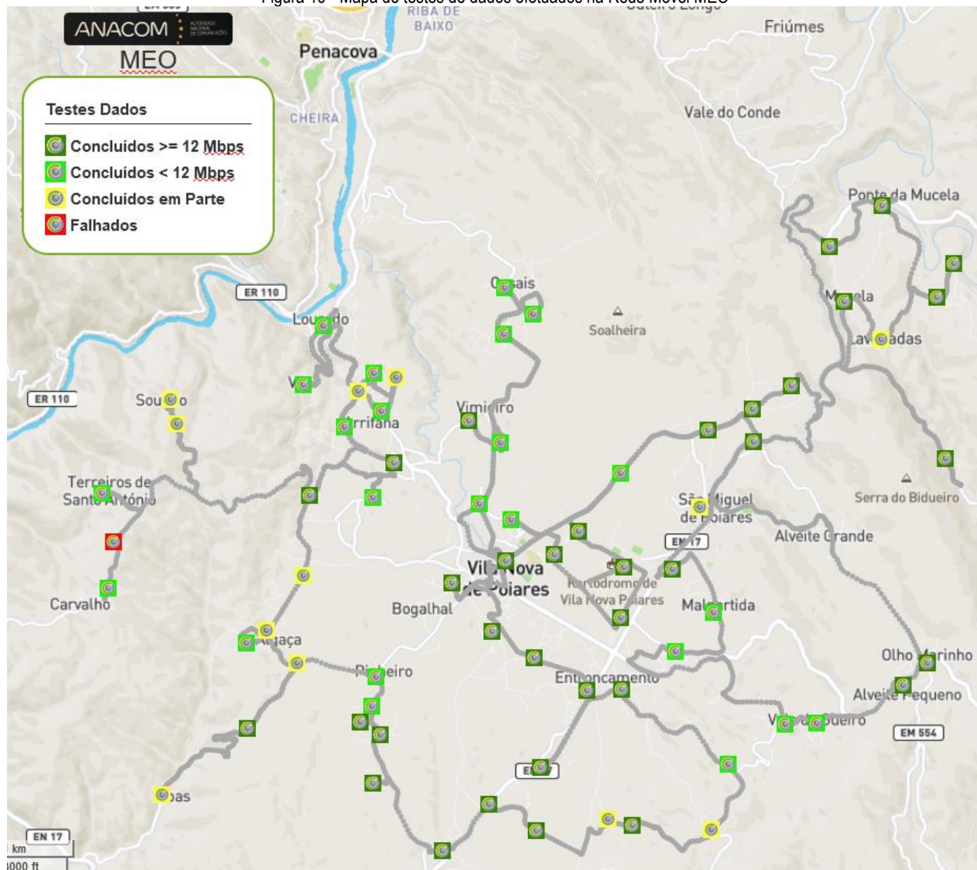
Figura 19 - Mapa de testes de dados efetuados na Rede Móvel MEO
