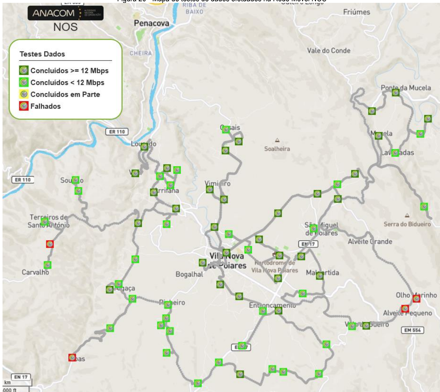
Figura 20 - Mapa de testes de dados efetuados na Rede Móvel NOS
