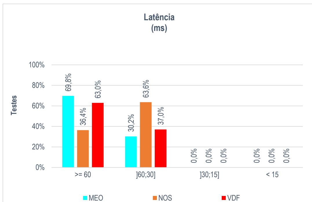
Figura 9 – Latência
