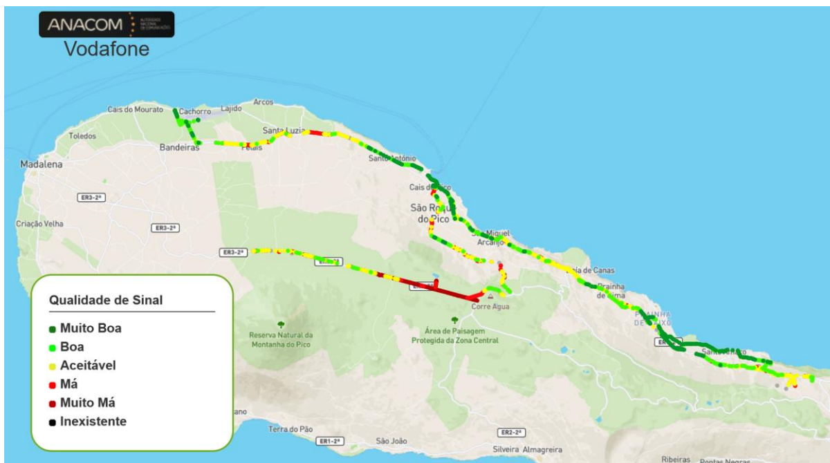
Figura 15 - Cobertura Móvel Vodafone (qualidade de sinal)
