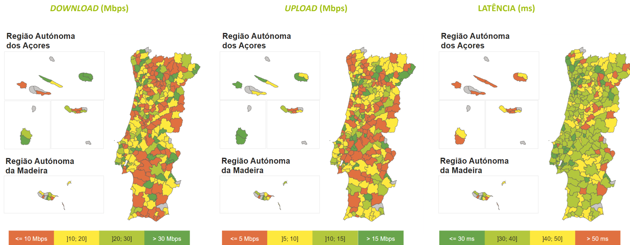
Figura 11 – Intervalos dos resultados medianos ( download , upload e latência) nos acessos móveis, por concelho de Portugal (3T2023)
