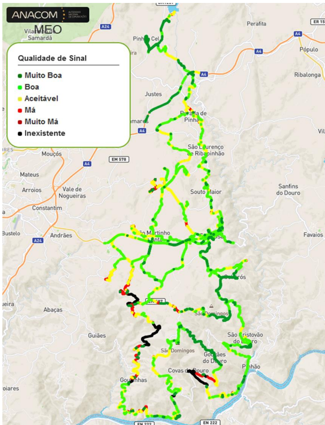
Figura 12 - Cobertura Rede Móvel MEO
