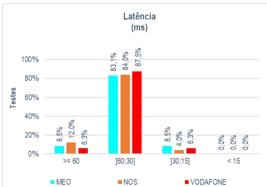
Figura 8 – Latência por Operador
