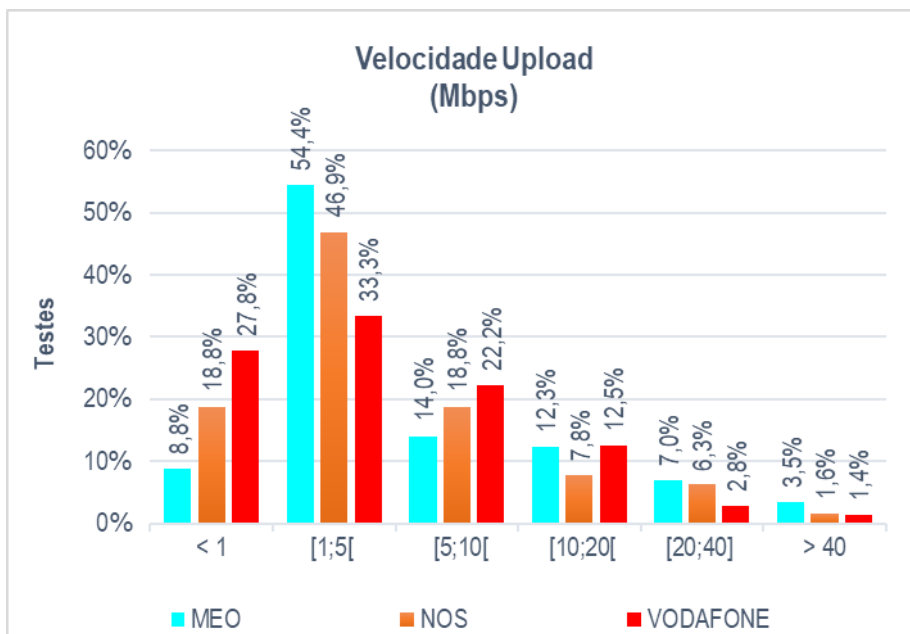
Figura 11 - Velocidade de Upload por Operador
