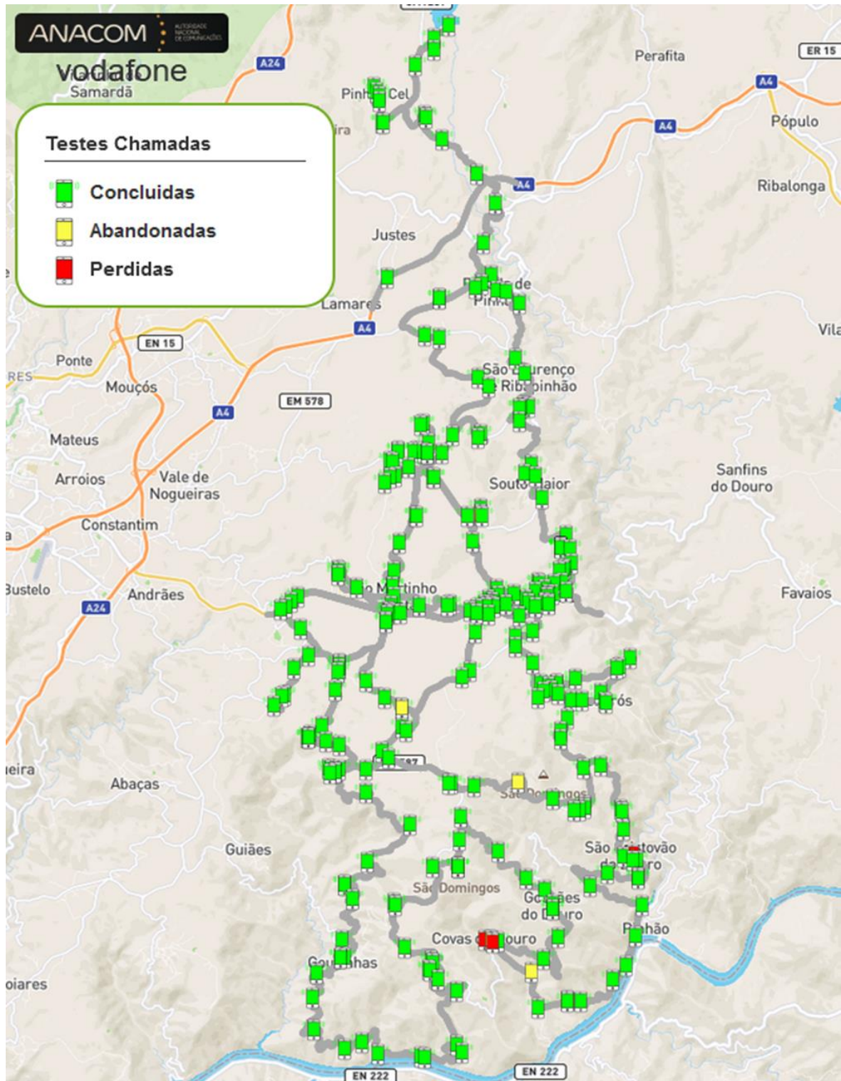
Figura 18 - Mapa de chamadas de voz efetuadas na Rede Móvel VODAFONE
