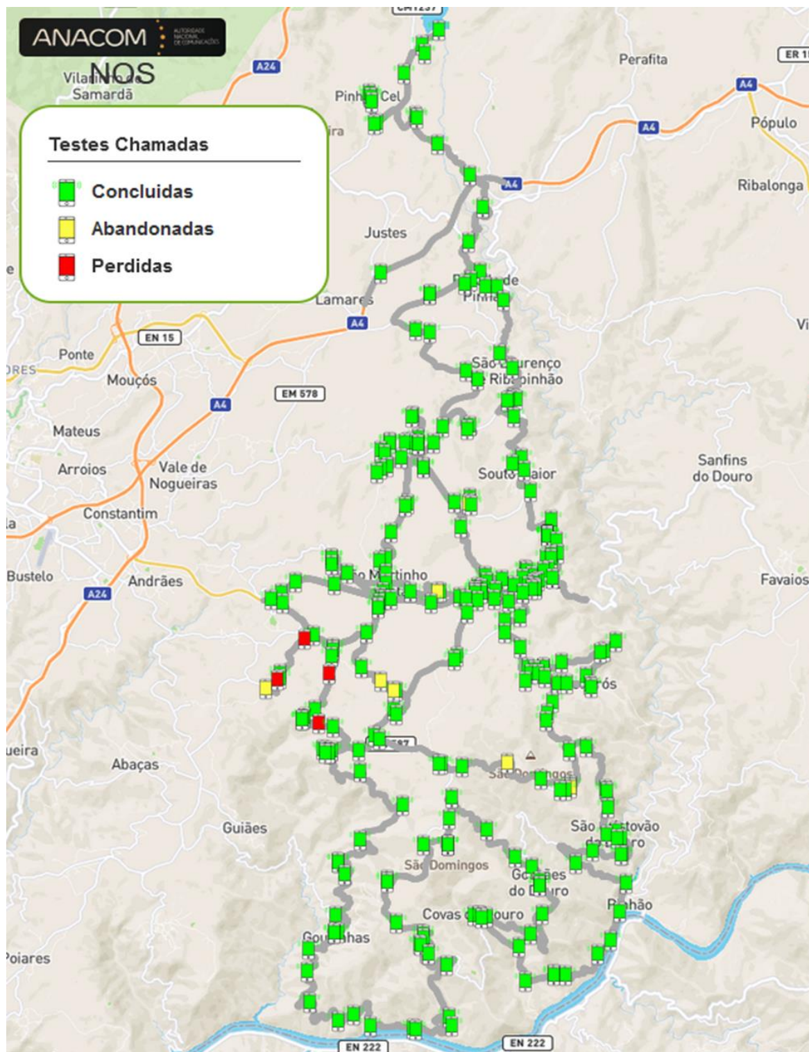
Figura 17 - Mapa de chamadas de voz efetuadas na Rede Móvel NOS
