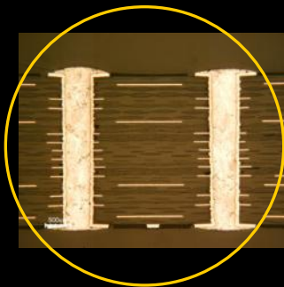
Corte de uma placa multicamada
