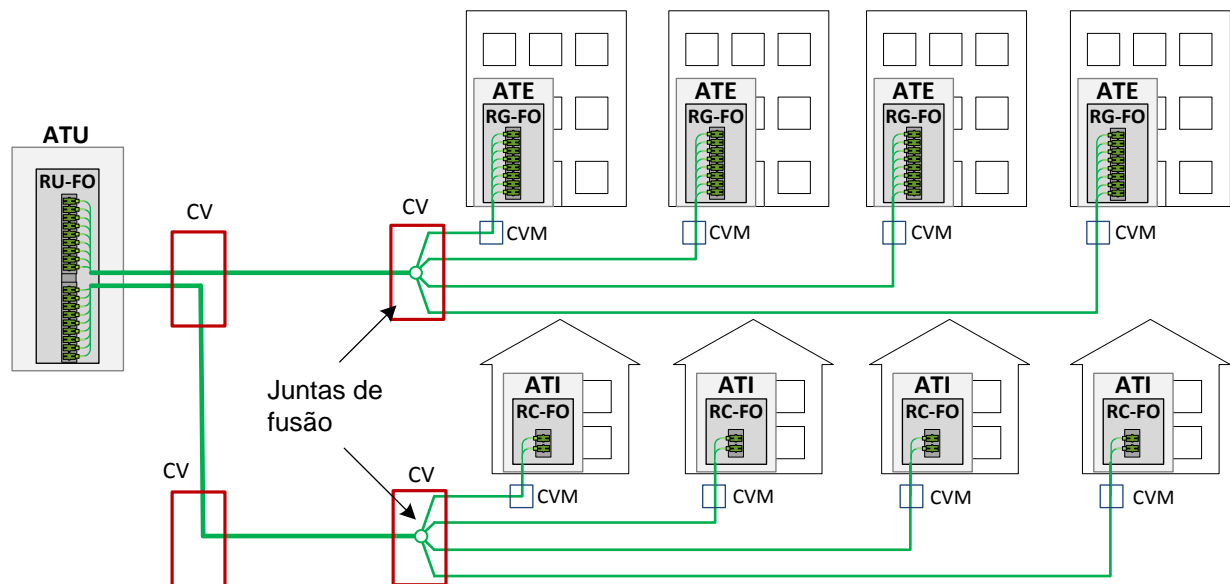
4.20 - Rede de Fibra Ótica da ITUR.
