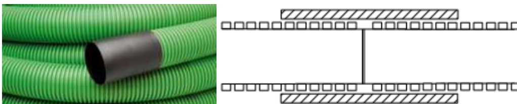
3.7 - União de tubo corrugado de dupla parede
