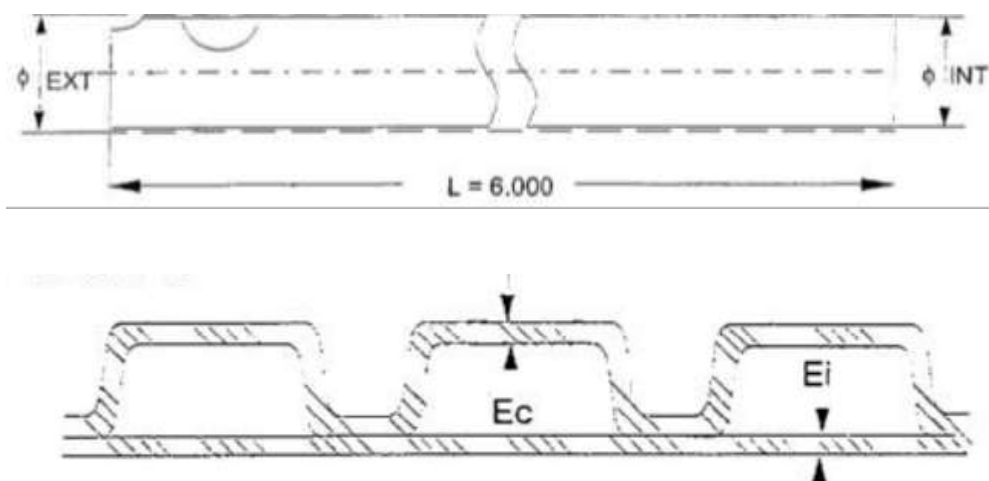
3.1 - Corte longitudinal de um tubo corrugado
