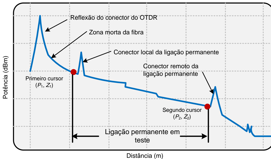
6.21 - Resultado do ensaio de reflectometria
