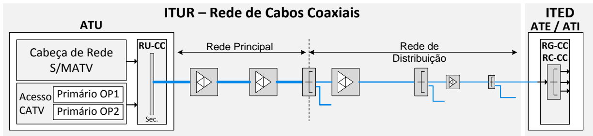
4.9 - troços constituintes da rede coaxial de uma ITUR.
