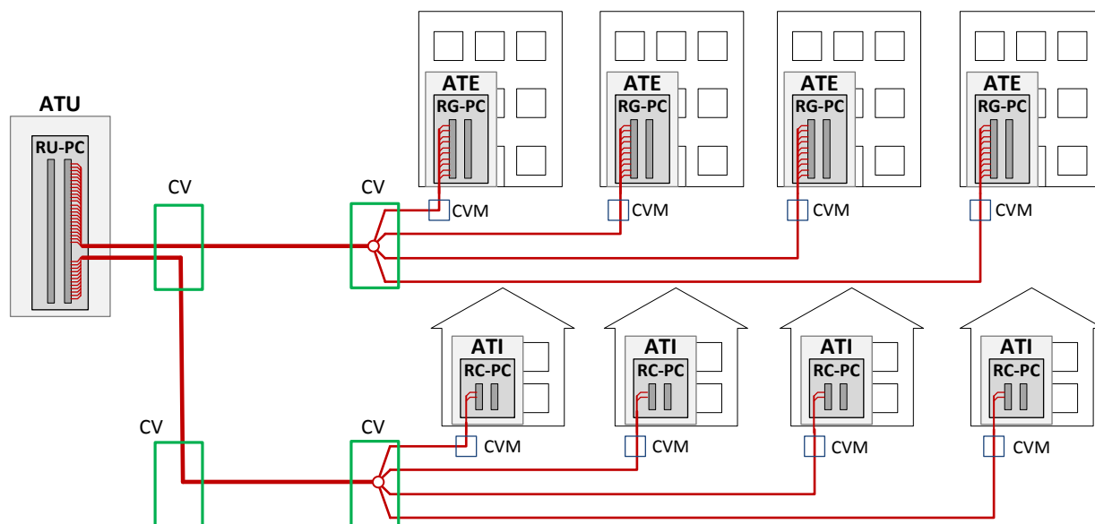
4.8 - Exemplo de rede de pares de cobre.
