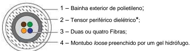
3.37 - Cabo de fibras óticas com estrutura monotubo
