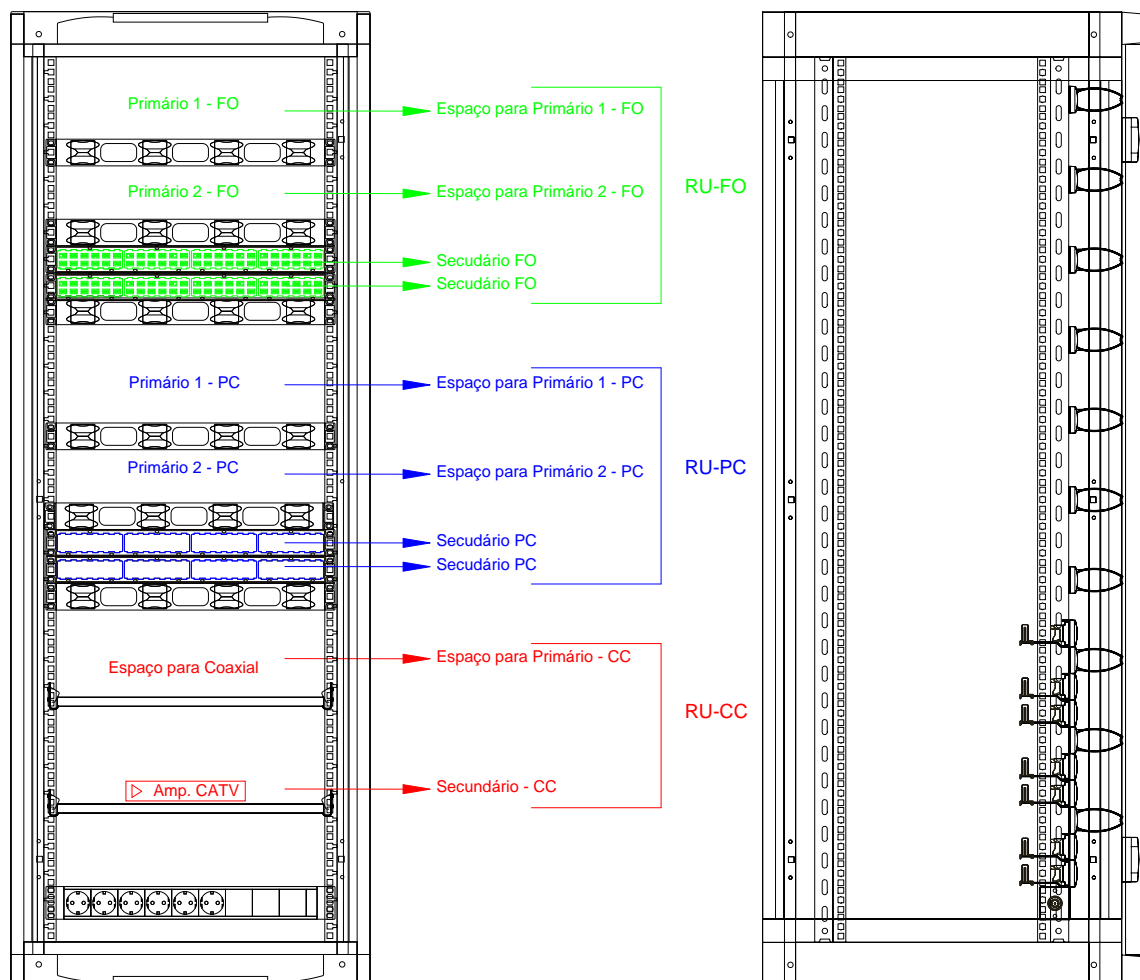
3.28 - Exemplos de armário de bastidor
