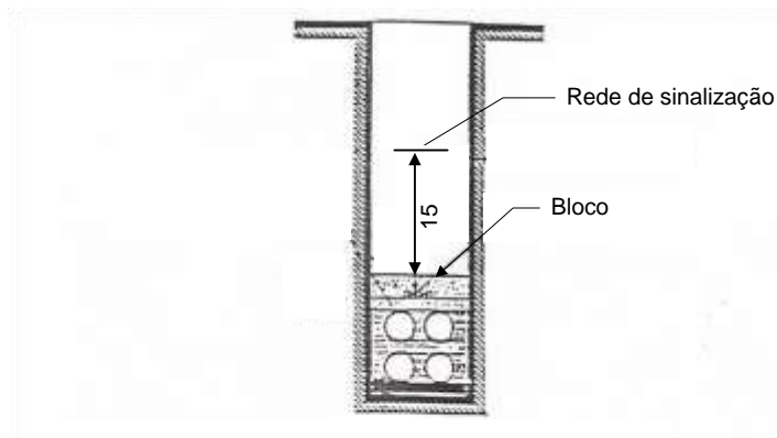
5.2 - Desenho esquemático de corte de uma vala técnica
