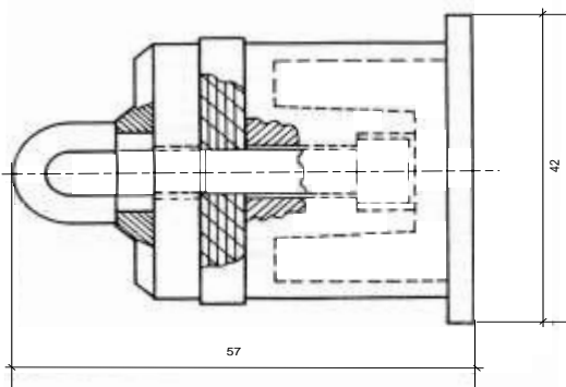
3.15 - Tampões tipo “fêmea” para tritubo PEAD
