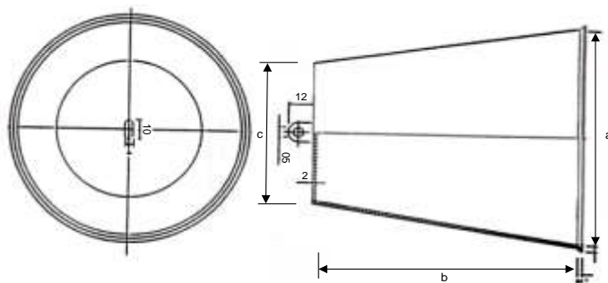
3.13 - Tampões para tubos corrugado de dupla face
