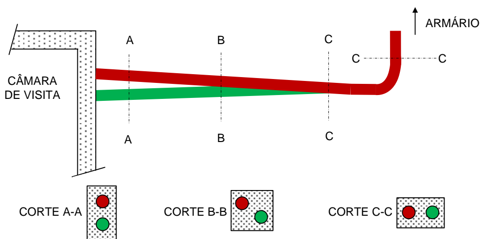
4.7 - Diagrama de entrada de tubos no pedestal
