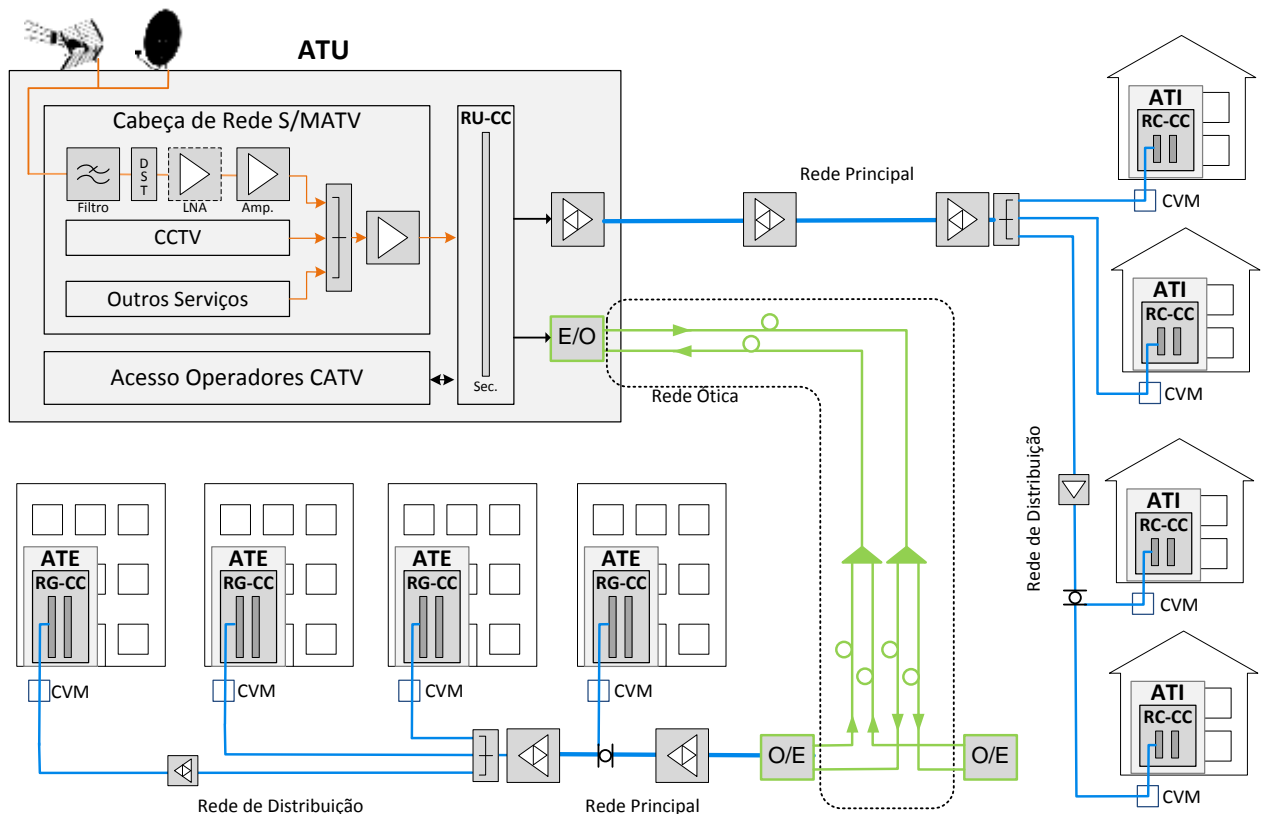
4.10 - Exemplo de arquitetura de uma rede híbrida de uma ITUR.
