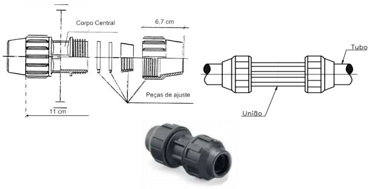
3.9 - União de tritubo através de uniões de aperto mecânico
