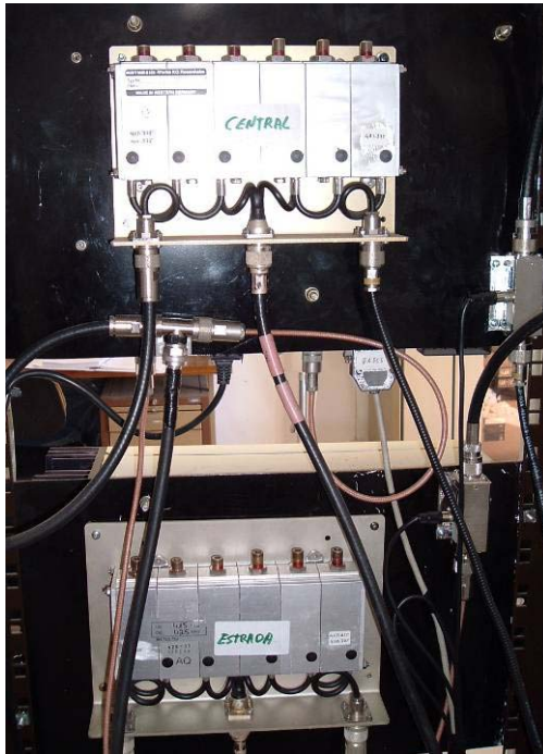
Figura 7. 'Multiplexers', combinadores de RF, e respectivos cabos coaxiais e conectores de um sistema de repetidores do Serviço Móvel Terrestre.
