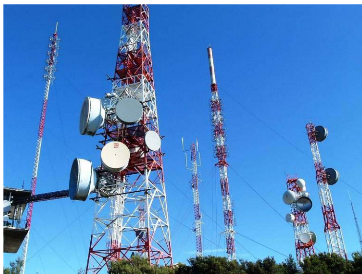
Figura 42. Elevado número de Fontes de RF num ‘site’ congestionado.
