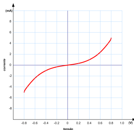
Figura 26. Característica i-v típica de uma junção Al- \text{Al}_2\text{O}_3 -Al.
