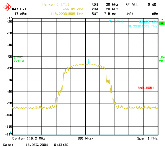
(a) (b) Figura 43. Monitorização do Espectro. (a) Análise Espectral. (b) Espectrograma.
