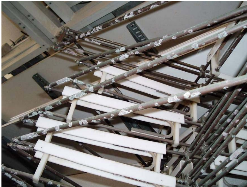
Figura 57. Sistema Radiante que originou o problema de interferências.
