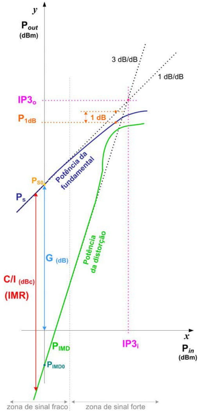
Figura 17. Interpretação gráfica do Ponto de Intersecção de 3.ª Ordem (IP3)
