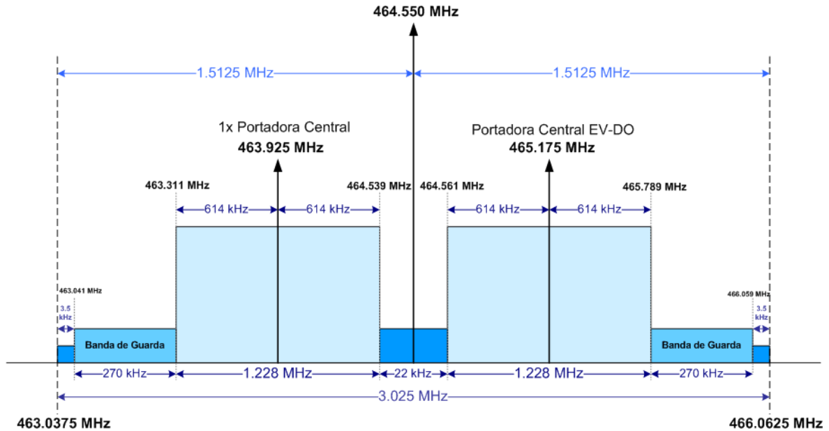
Figura 60. Máscara espectral do DL do sistema CDMA 450.
